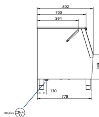
VISTA LATERALE SIDE VIEW - VUE LATÉRALE - VISTA LATERAL
