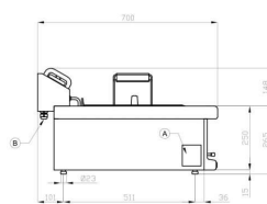
A - Targhetta caratteristiche B - Allacciamento elettrico
