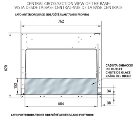
VISTA DELLA BASE DALLA ZONA CENTRALE CENTRAL CROSS SECTION VIEW OF THE BASE VISTA DESDE LA BASE CENTRAL - VUE DE LA BASE CENTRALE
