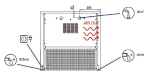
VISTA POSTERIORE REAR VIEW - VUE ARRIERE - VISTA TRASERA
