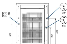
VISTA POSTERIORE REAR VIEW - VUE ARRIERE - VISTA TRASERA
