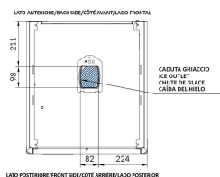
VISTA DELLA BASE DALLA ZONA CENTRALE CENTRAL CROSS SECTION VIEW OF THE BASE: VISTA DESDE LA BASE CENTRAL-VUE DE LA BASE CENTRALE
