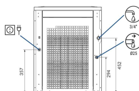
VISTA POSTERIORE REAR VIEW - VUE ARRIERE - VISTA TRASERA
