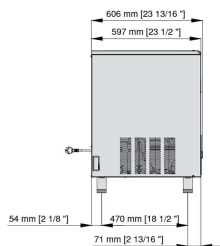
VISTA LATERALE
