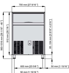
VISTA FRONTALE
