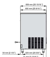
VISTA LATERALE
