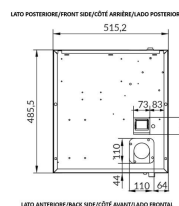
VISTA DELLA BASE DALLA ZONA CENTRALE CENTRAL CROSS SECTION VIEW OF THE BASE - VISTA DESDE LA BASE CENTRAL VUE DE LA BASE CENTRALE
