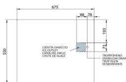
VISTA DELLA BASE DALLA ZONA CENTRALE CENTRAL CROSS SECTION VIEW OF THE BASE VISTA DESDE LA BASE CENTRAL-VUE DE LA BASE CENTRALE
